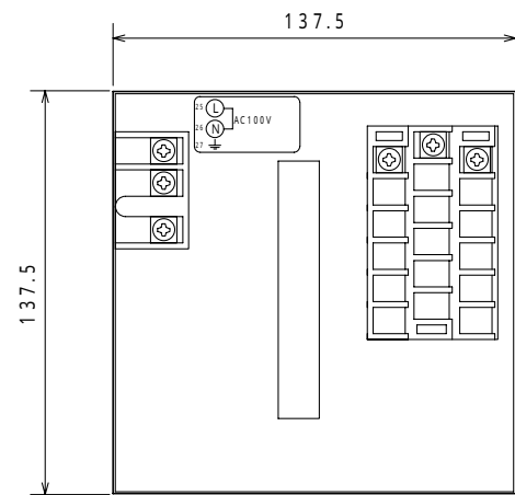
端子台図
